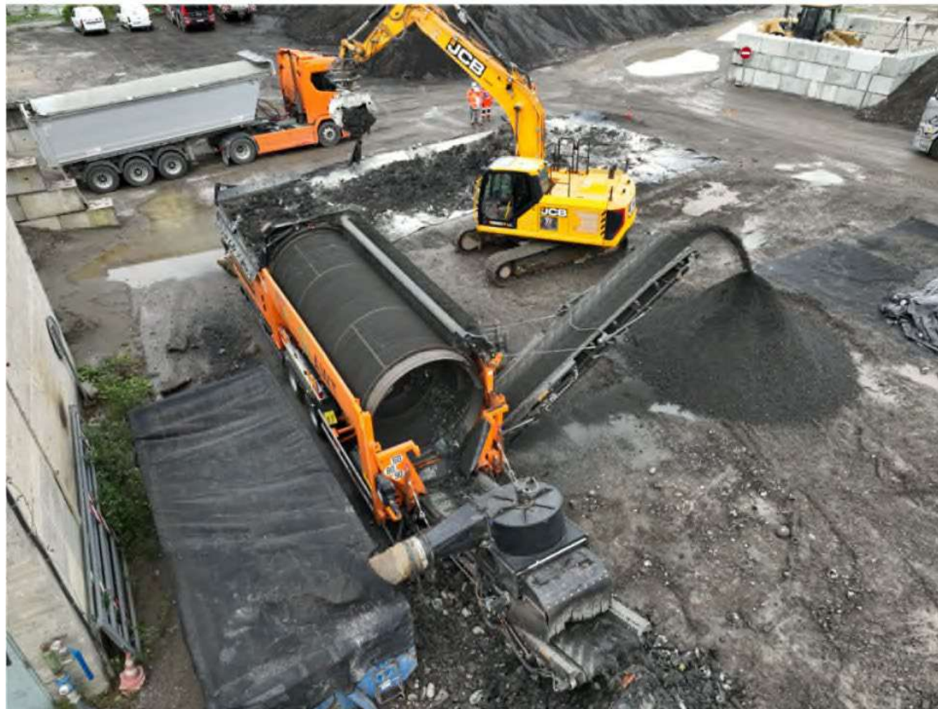
Exemple d'un Cribleur rotatif
